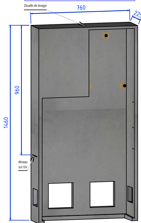
SARCOTECH S20 DROIT / SOCLE DOUBLE
